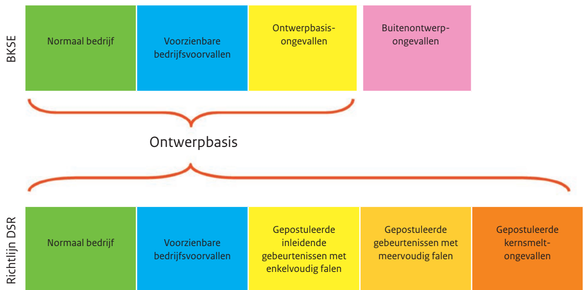
Figuur 1: Vereenvoudigde weergave van de ontwerpbasis volgens het Bkse en de Handreiking VOBK.
