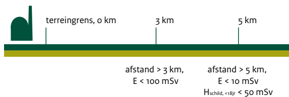
Figuur 2: Zones en interventiewaarden bij gepostuleerde kernsmeltongevallen.
